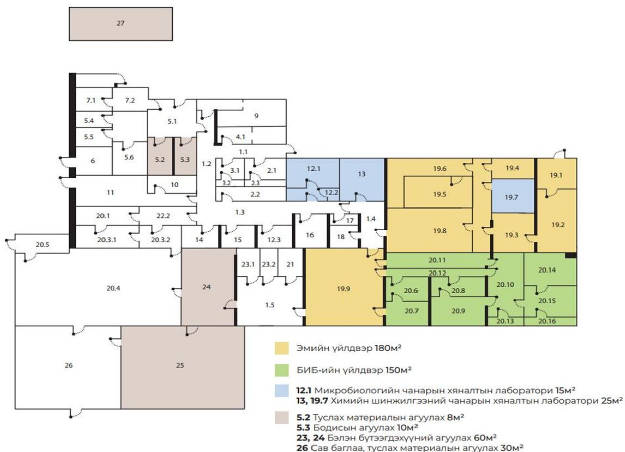
Зураг 1. Монхимо үйлдвэрийн цогцолборын план зураг
