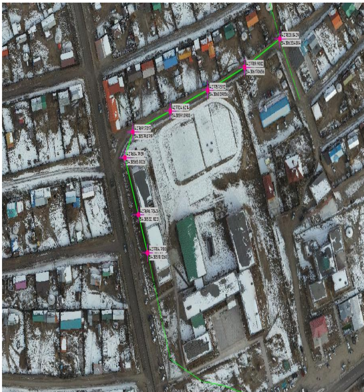
Зураг 7. Наран багийг бохирын шугамд холбох байршил
