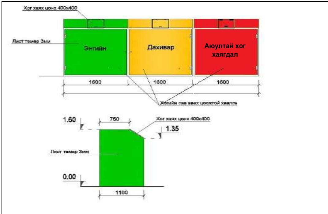
Зураг 5.1. Хог хаягдлын цэгийн шийдэл
