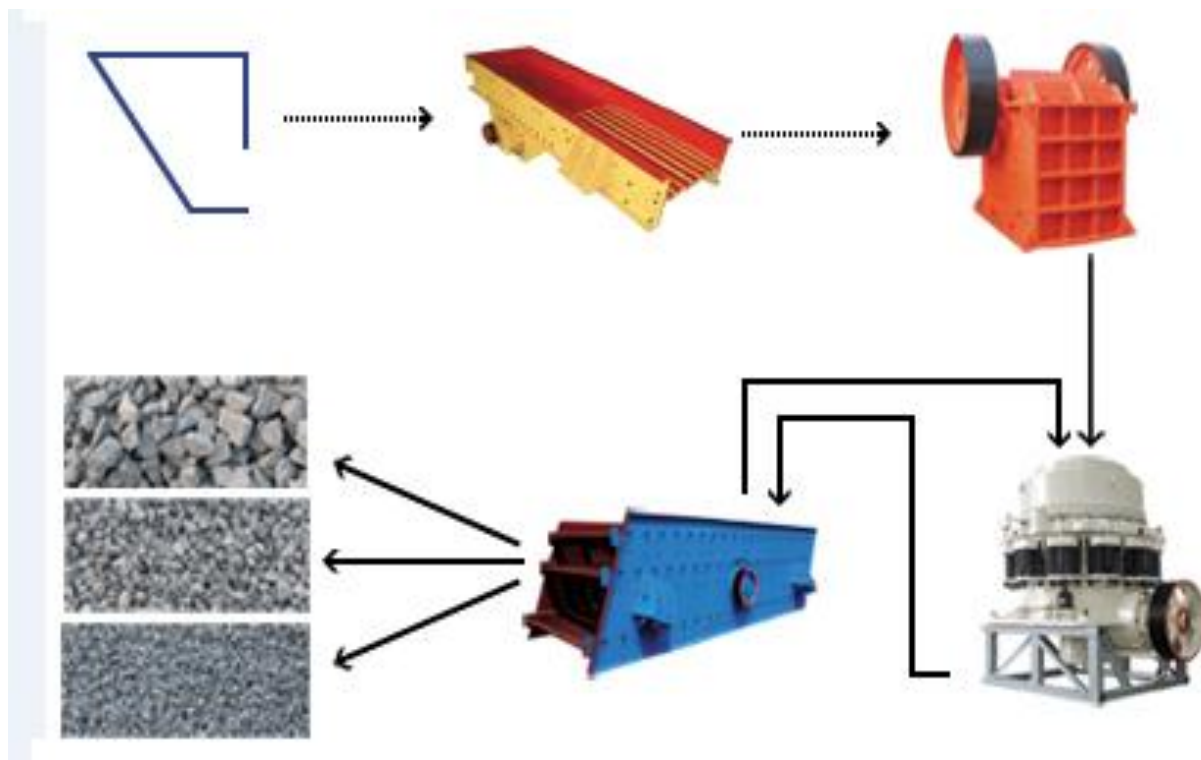
Зураг 3. Бутлах цехийн тоног төхөөрөмжийн холболтын схем
