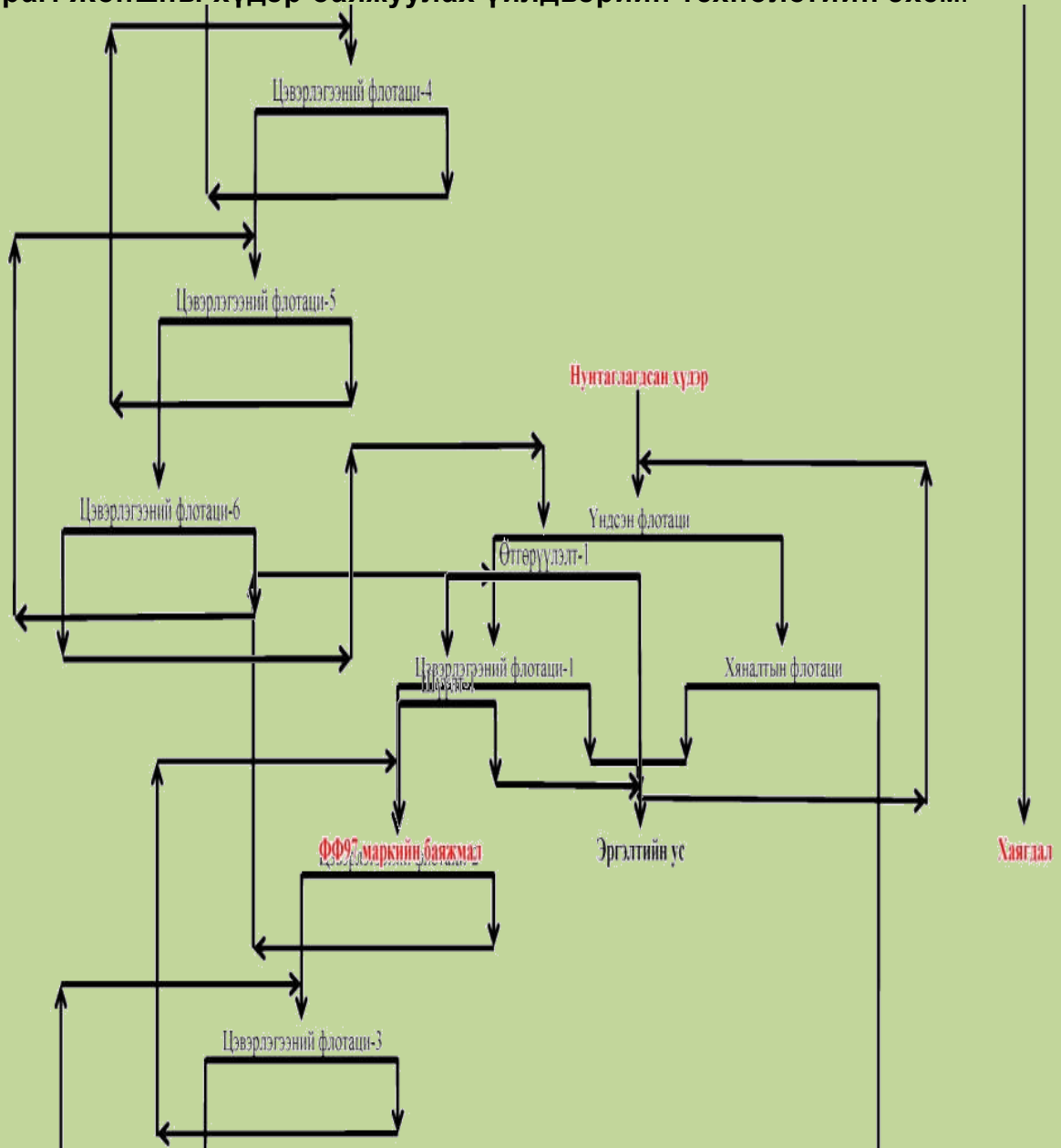
2 –р зураг. Жоншны хүдэр баяжуулах үйлдвэрийн технологийн схем.
