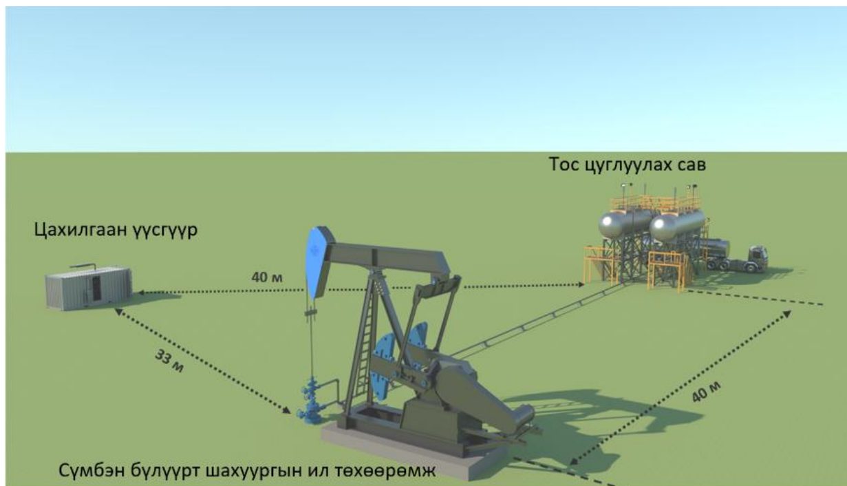
Зураг 1.10. Дан цооноогоор олборлох систем
