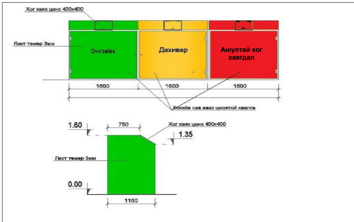
Зураг 1.5 Хог хаягдлын цэгийн шийдэл
