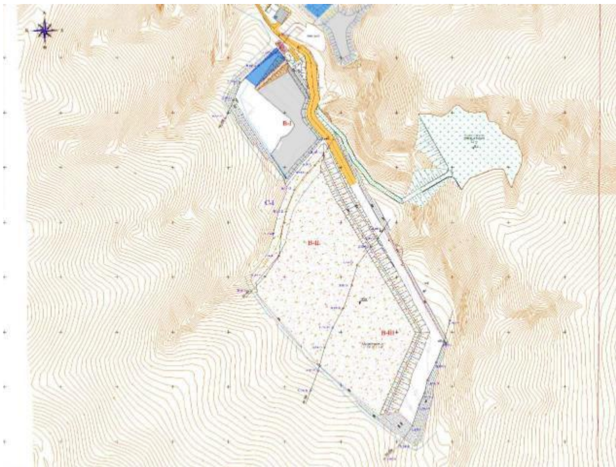
Зураг 4. Ил уурхайн ашиглалтын эцсийн байдал
