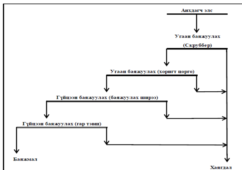
Зураг 6. Элсийг угаах технологийн ерөнхий схем
