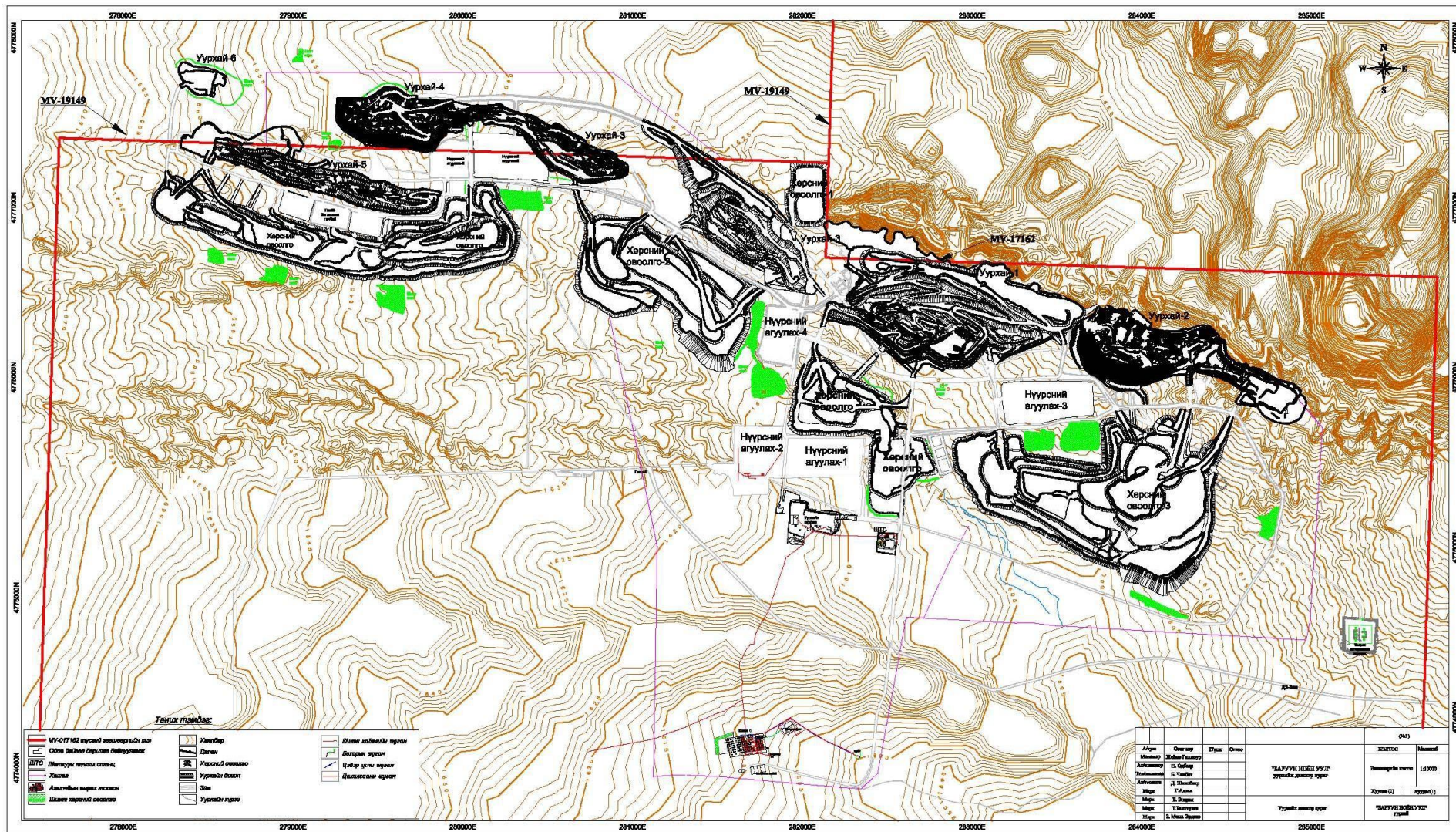
Уурхайн ерөнхий план зураг
