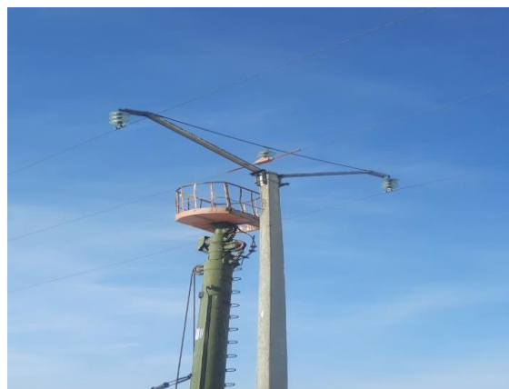
Зураг 9.3ТБ-18 , СВ-11 маркийн төмөр бетонон дундын тулгуурт шувуу хамгаалах полимер суурилуулсан байдал
