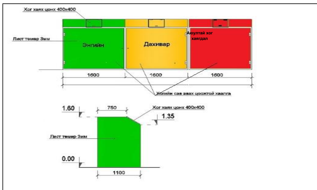
Зураг 10. Хог хаягдлын цэгийн шийдэл
