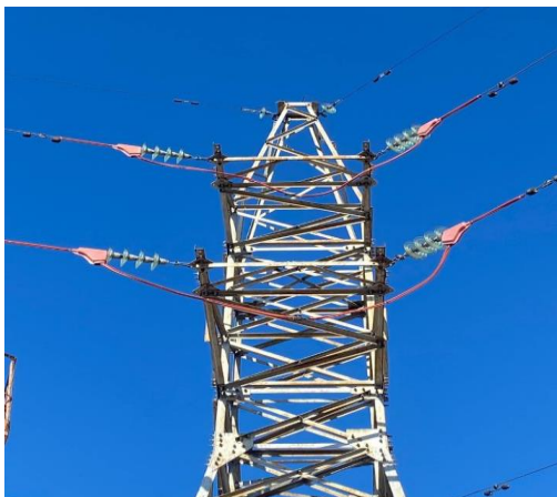
Зураг 7.У-35 2Т маркийн төмөр анкер болон СВ-15 маркийн төмөр бетонон анкерт шувуу хамгаалах полимер суурилуулсан байдал.
