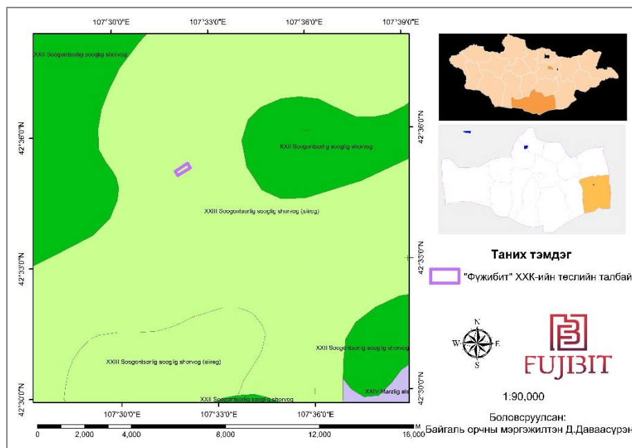
Зураг 15. Төслийн талбай орчмын ургамлан нөмрөг
