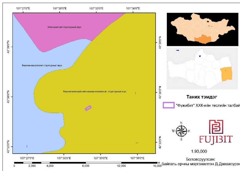
Зураг 12. Төслийн талбай орчмын геологийн тогтоц
