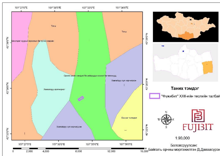
Зураг 11. Төслийн талбай орчмын геоморфологи
