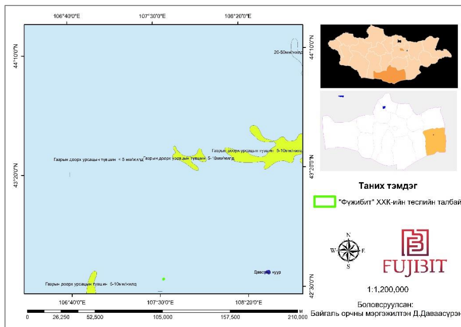
Зураг 13. Төслийн талбай орчмын газрын доорх усны нөхөн сэргээгддэг нөөцийн тархалт
