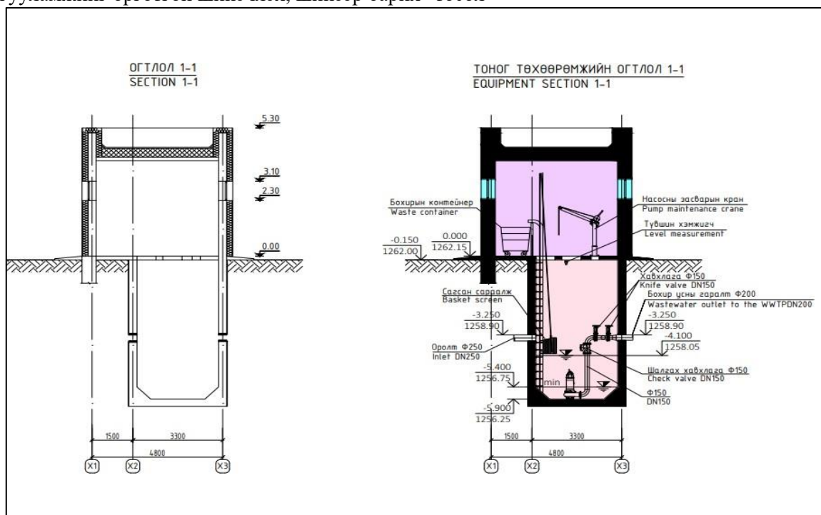
Зураг 7. Хотын төвд төлөвлөж шинэ насос станцын технологийн зураг
