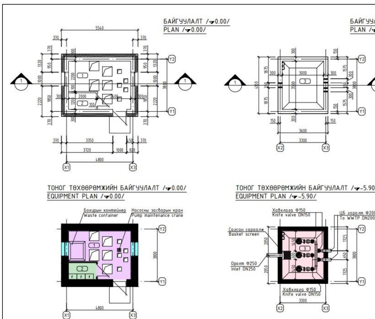
Зураг 6. Хотын төвд төлөвлөж шинэ насос станцын байр зүйн зураг
