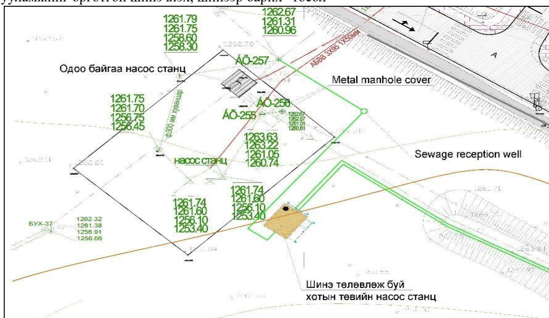
Зураг 6. Хотын төвд төлөвлөж шинэ насос станцын байр зүйн зураг
