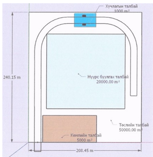
Зураг 1. Талбайн ерөнхий төлөвлөгөөний зураг
