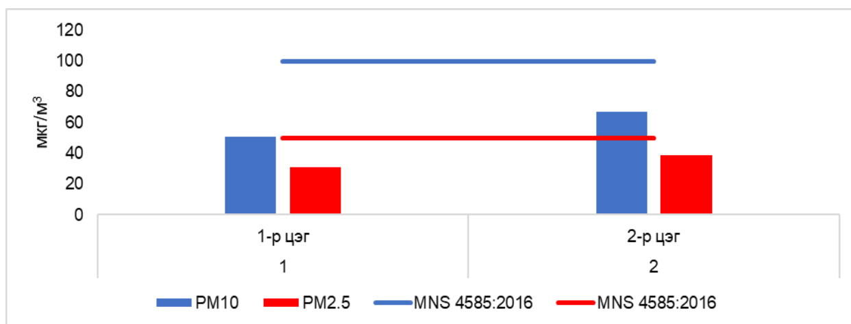
График 1. Том болон нарийн ширхэглэгт тоосонцрын хэмжилтийн утга
