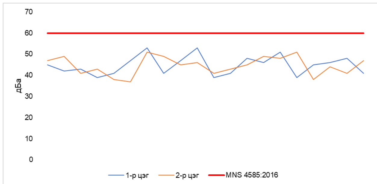
График 3. Дуу шуугианы хэмжилтийн утга
