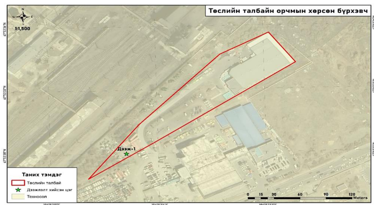
Зураг 6. Хөрсөн бүрхэвчийн тархалт
