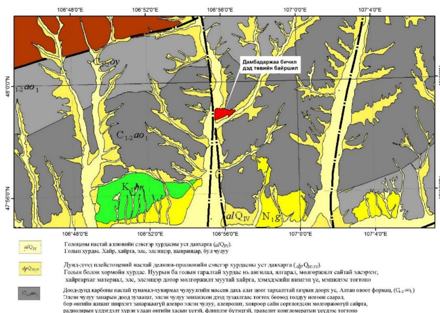
Зураг 3-2. Төслийн талбай орчмын геологи
