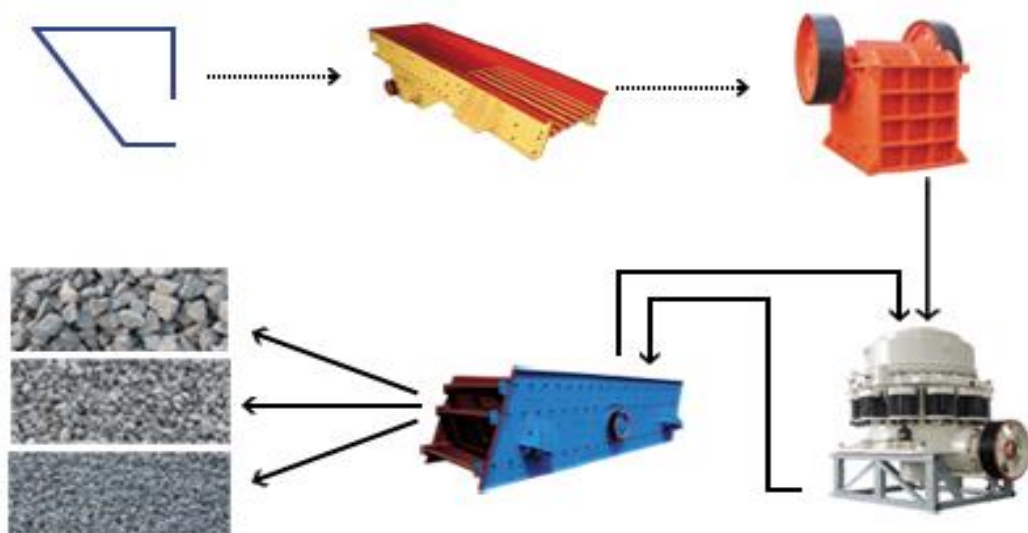
Зураг 2. Тоног төхөөрөмжийн дамжлагын схем
