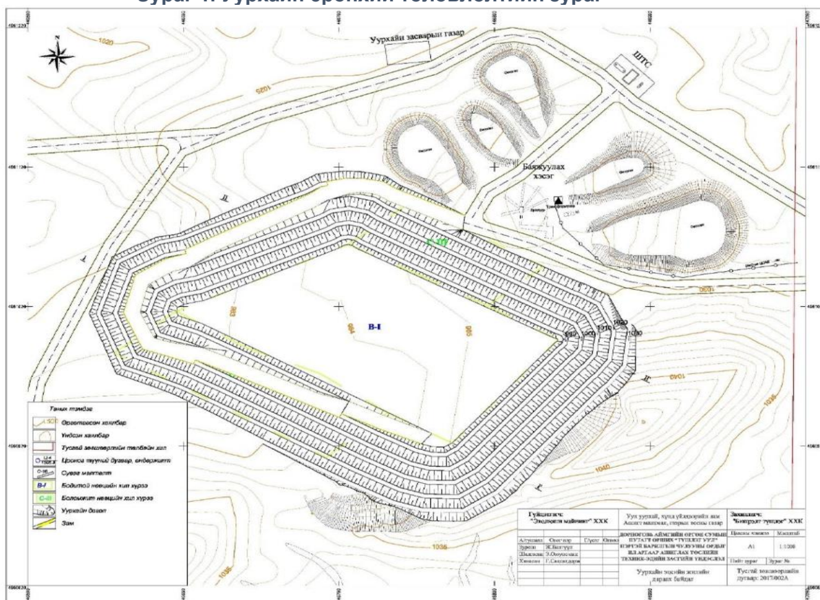
Зураг 1. Уурхайн ерөнхий төлөвлөлтийн зураг
