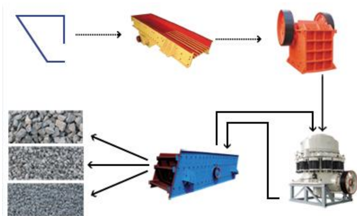
Зураг 2. Бутлан ангилах хэсгийн дамжлагын схем зураг
