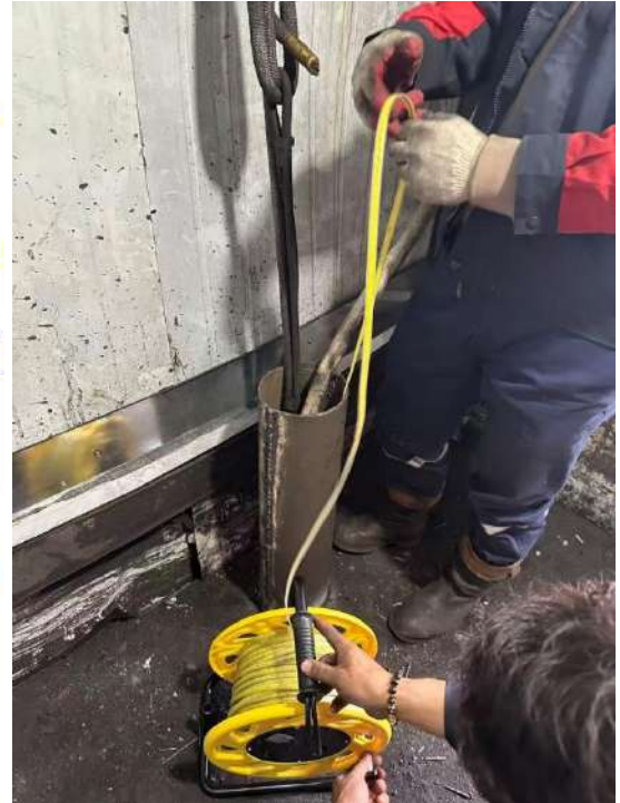
Зураг № 40 Усны түвшин хэмжилт
