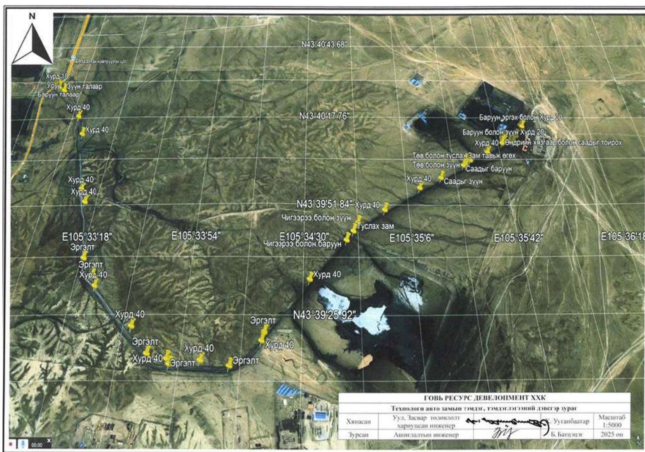
Зураг №7 Нэмэлтээр байрлуулах тэмдэгний төлөвлөгөө
