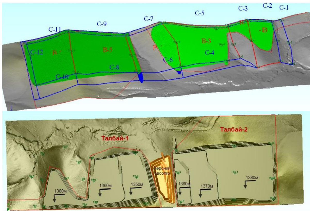
Зураг 1. Морин уулын өмнөд хэсгийн барилгын чулууны ордын нөөцийн блок модель ба . Ил уурхайн ерөнхий загварчлал /Ашиглалтын эцсийн жил
