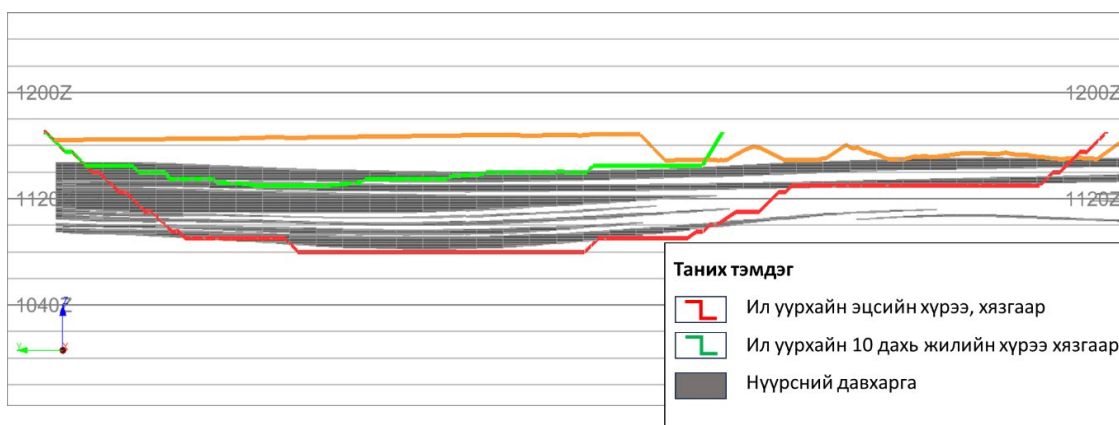
Зураг 8. Ил уурхайн уулын ажлын ахилт, (Зүсэлт А-А')
