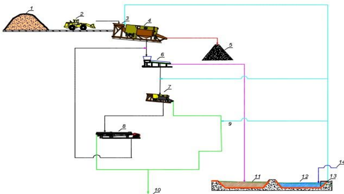
Зураг 6. Баяжуулах технологийн тоног төхөөрөмжийн холболтын схем
