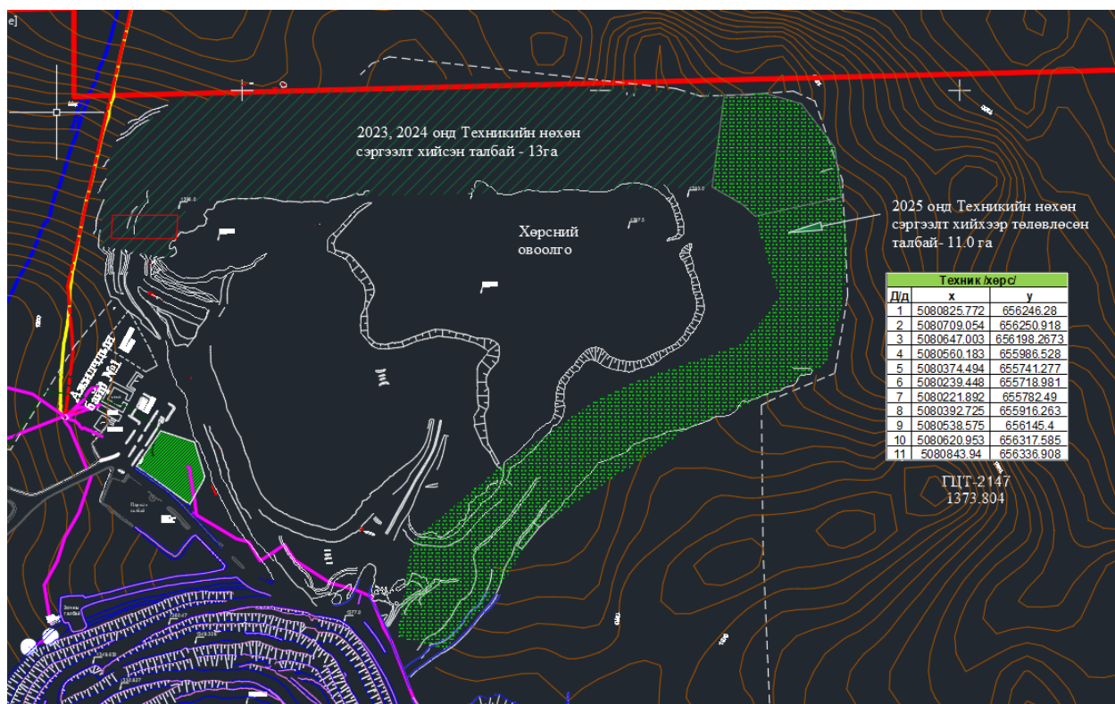
Зураг 1. Хөрсний овоолгын 2025 онд хийгдэх техникийн нөхөн сэргээлтийн зураг
