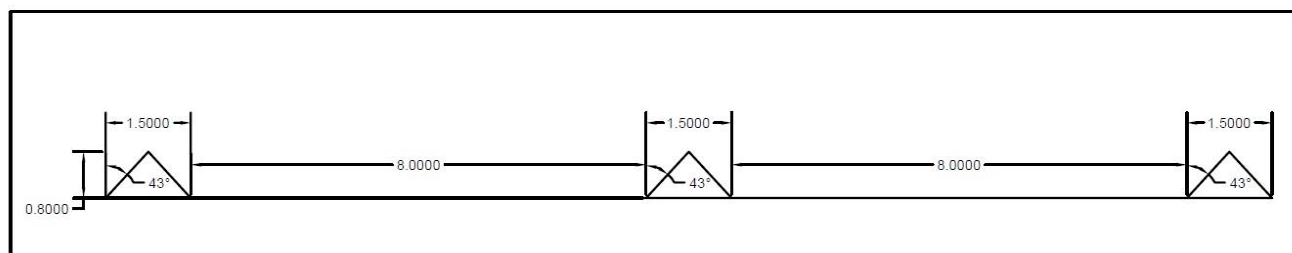
Зураг-3. Хаягдал хөрсний овоолгын хөндлөн огтлол
