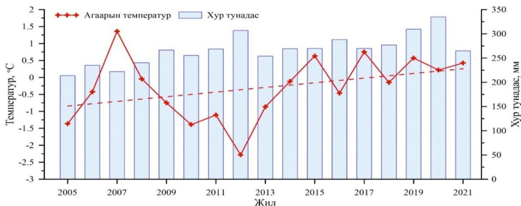
Зураг 36. Агаарын температур болон хур тунадасны олон жилийн хандлага
