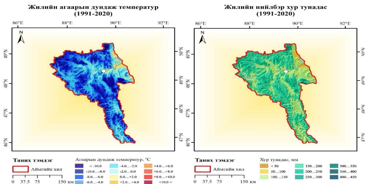
Зураг 35. Агаарын жилийн дундаж температур, жилийн нийлбэр хур тунадас (Эх сурвалж: www.irimhe.natem.gov.mn/ )
