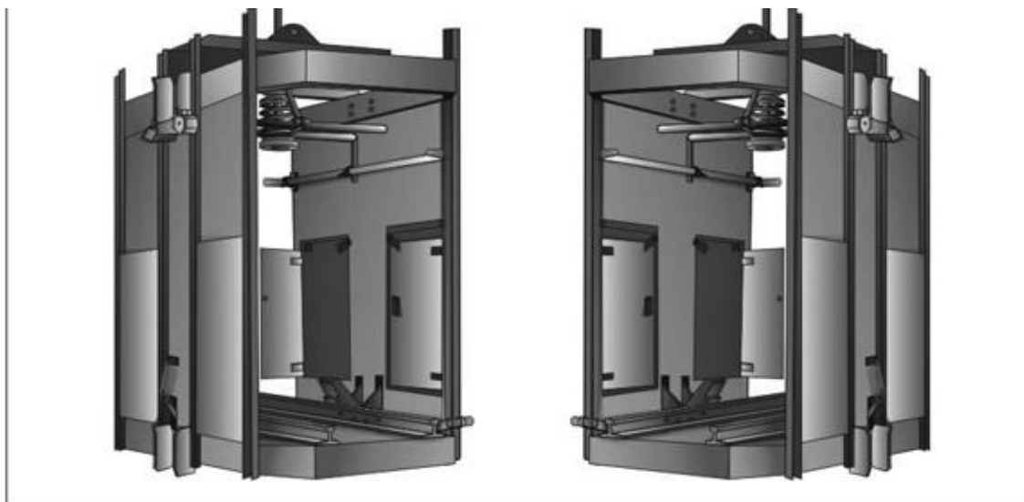
Зураг 21. 1KH1.4-1 маркийн далд уурхайн клет
