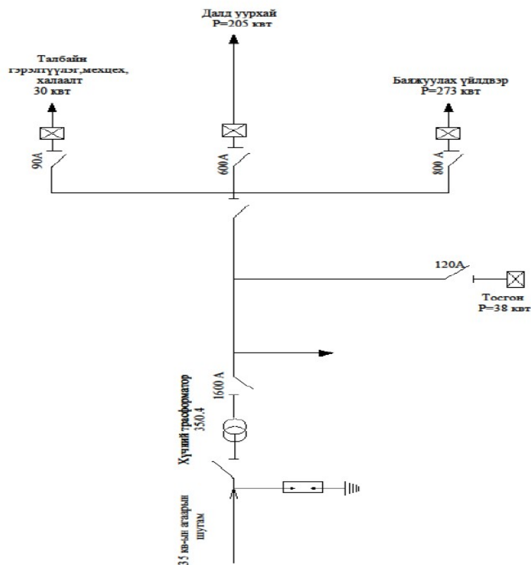
Зураг 8. Цахилгаан хангамжийн тойм схем
