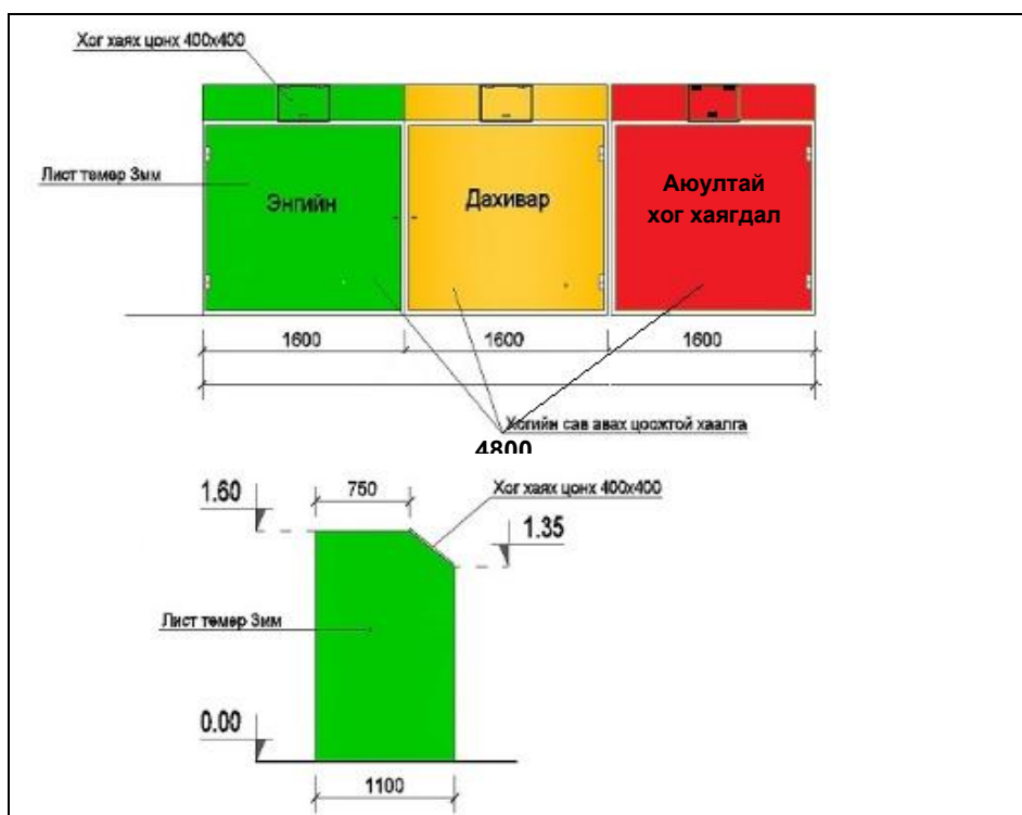
Зураг 5. Хог хаягдлын цэгийн шийдэл
