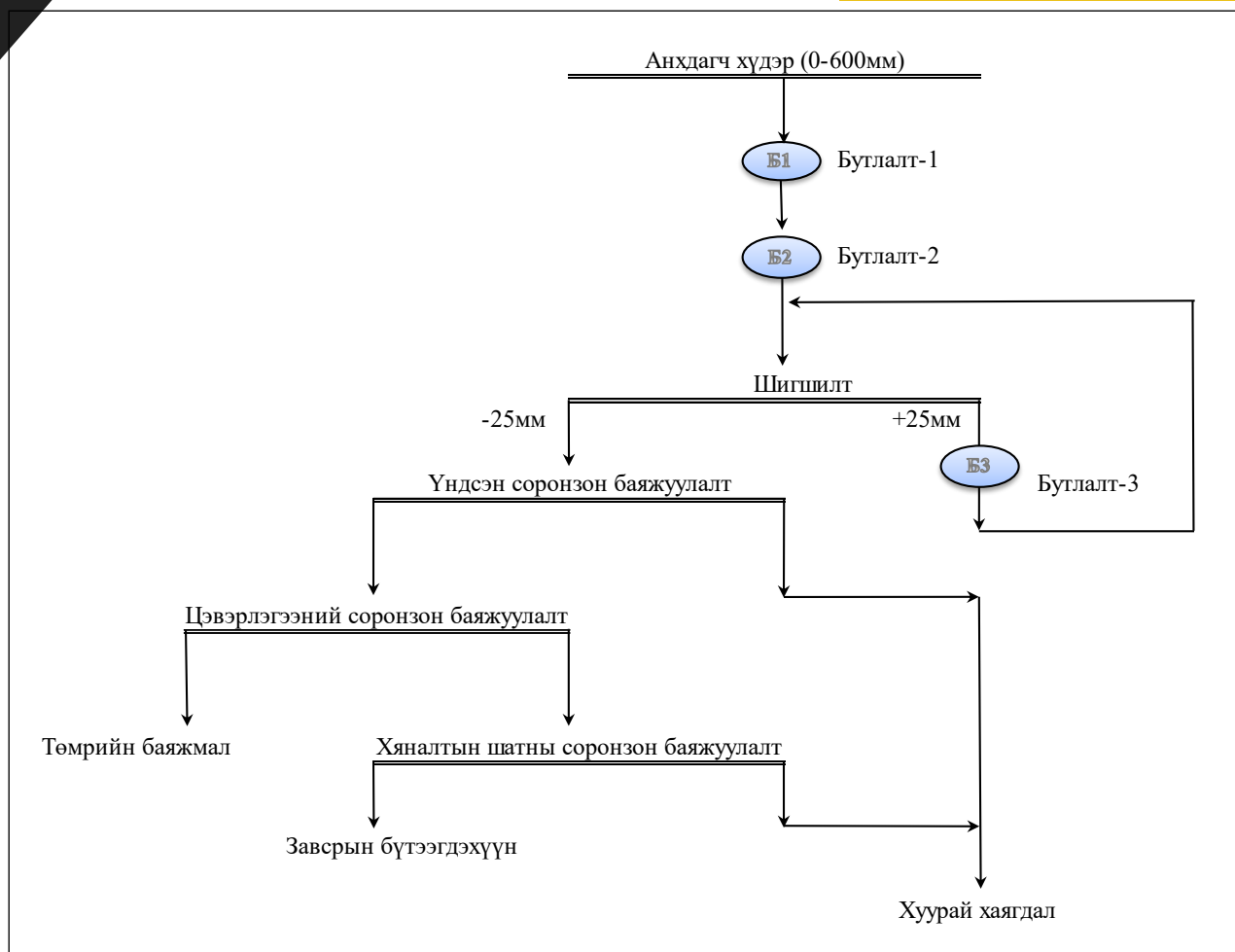
1-р зураг. Төмрийн хүдэр хуурай соронзон аргаар баяжуулах технологийн схем
