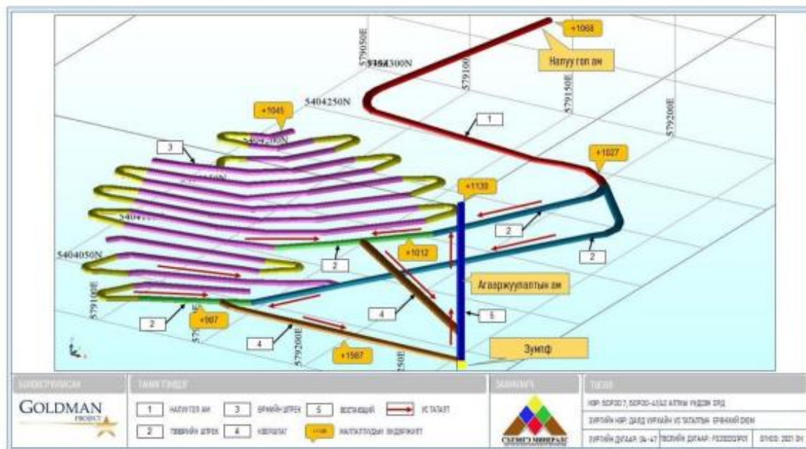
Зураг 15. Ус таталтын ерөнхий схем
