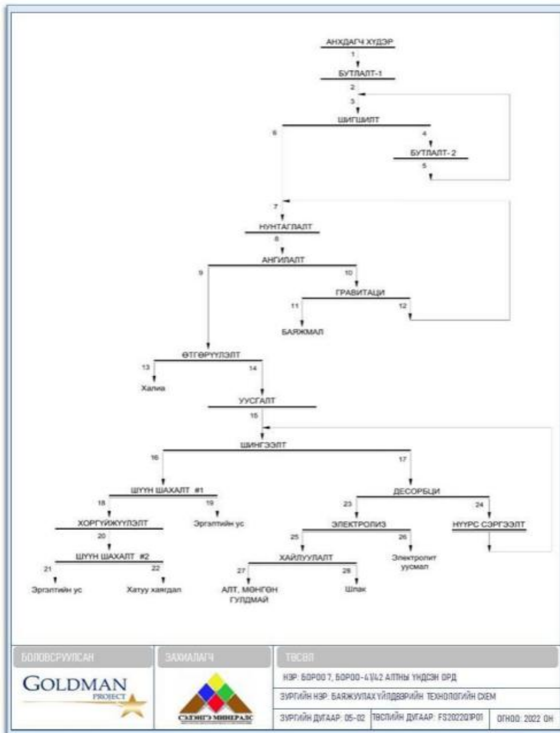
Зураг 14. Баяжуулах үйлдвэрийн технологийн схем
