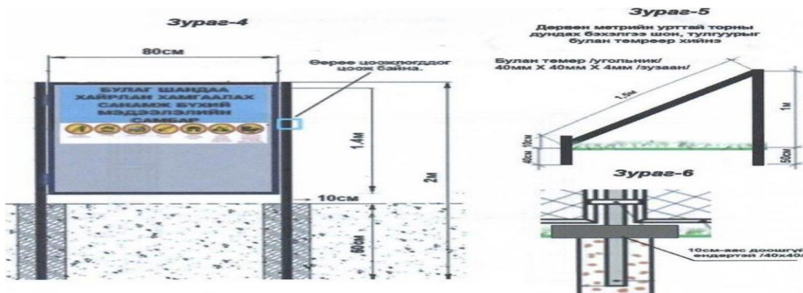
Зураг 19. Хун орж гарах хаалга, мэдээллийн самбар, бэхэлгээ
