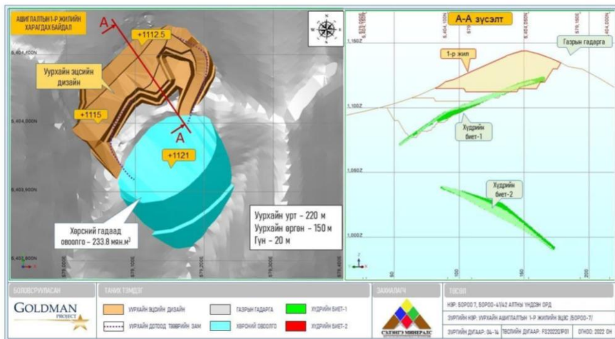
Зураг 5. Уурхайн ашиглалтын 1-р жилийн эцсийн харагдах байдал
