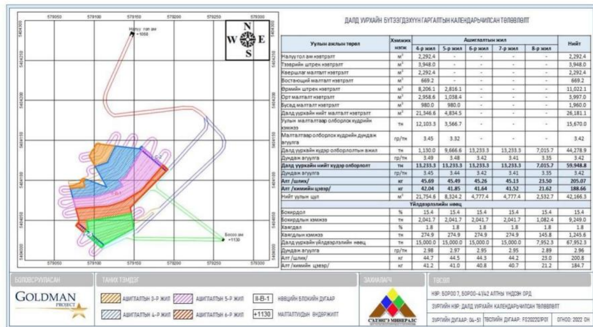
Зураг 13. Далд уурхайн календарьчилсан төлөвлөлт
