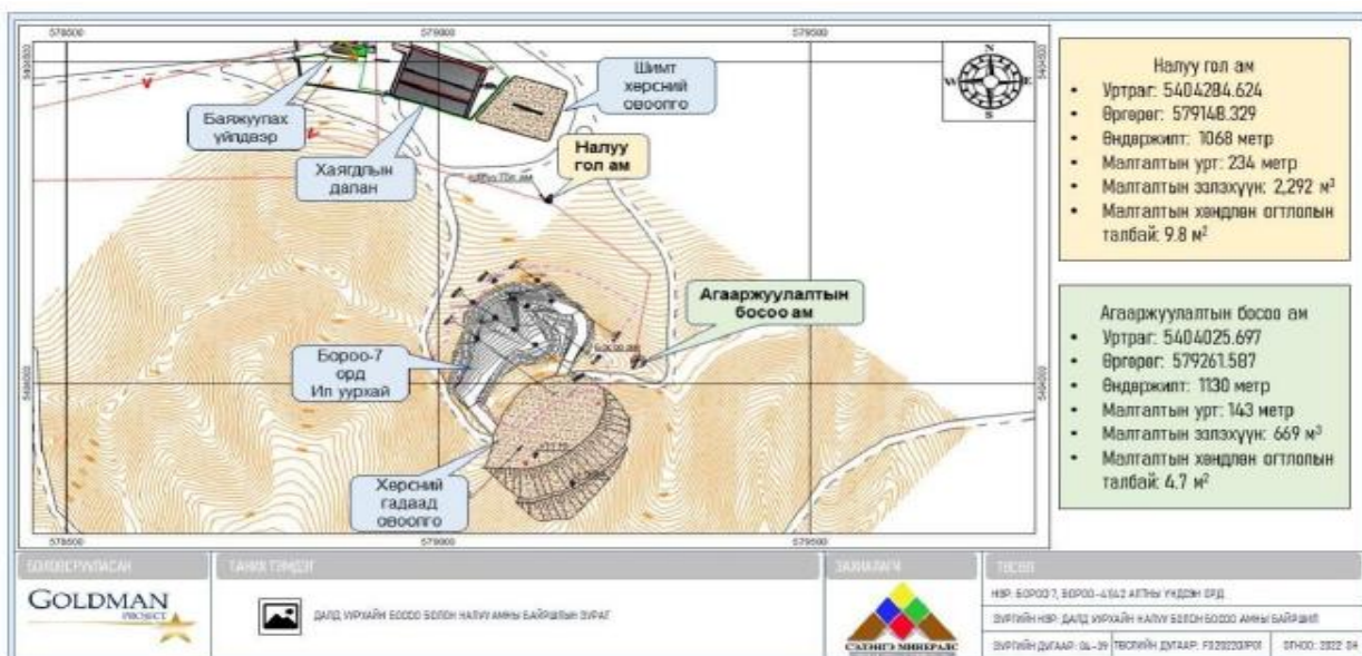
Зураг 10. Далд уурхайн налуу болон босоо амнуудын байршлын зураг
