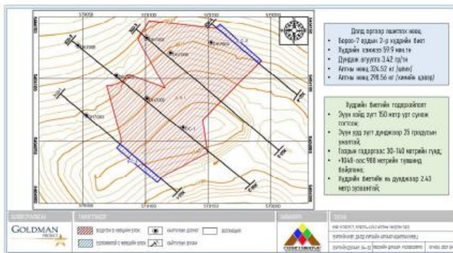
Зураг 8. Далд уурхайн аргаар ашиглах нөөц
