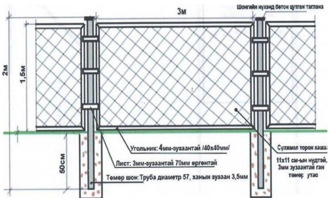
Зураг 18. Хамгаалах булагт орох материалын хэмжээ хийцийн схем зураг.
