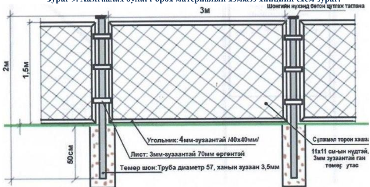
Зураг 9. Хамгаалах булагт орох материалын хэмжээ хийцийн схем зураг.
