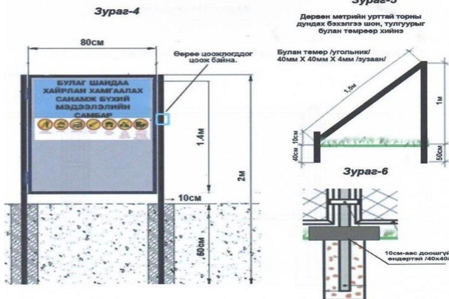
Зураг 10. Хун орж гарах хаалга, мэдээллийн самбар, бэхэлгээ
