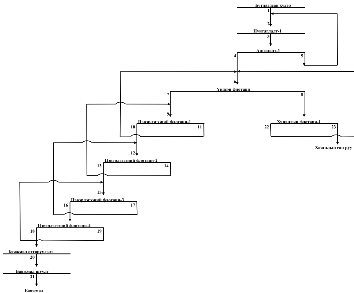
Зураг 3. Хүдэр флотацийн аргаар баяжуулах технологийн схем
