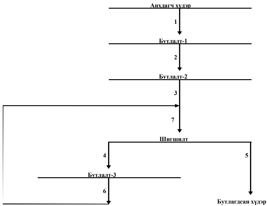
Зураг 2. Хүдэр бэлтгэлийн технологийн схем
