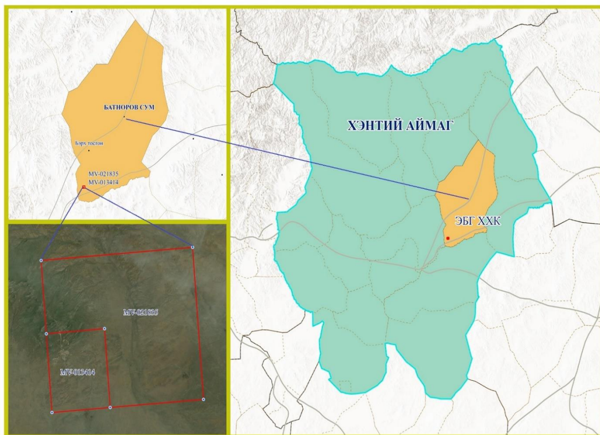
Зураг 1. “Идэрмэг 1, Идэрмэг 2” нэртэй хайлуур жоншны ордын байршлын зураг
