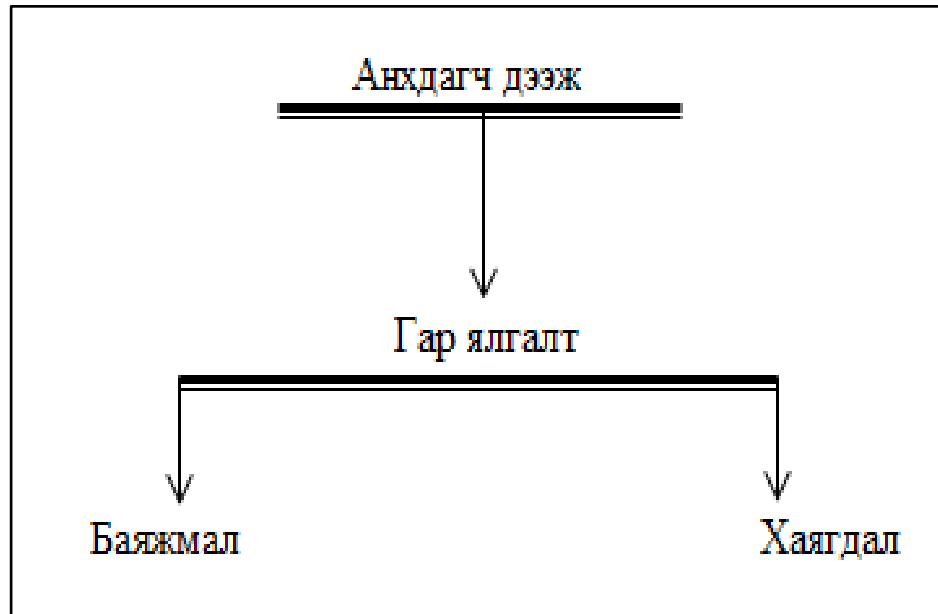
Зураг 3. Гар ялгалтын баяжуулалтын схем
