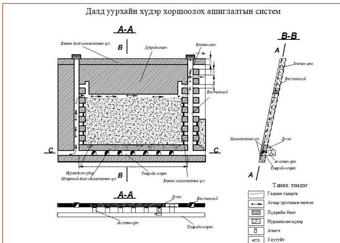
Зураг 2. Далд уурхайн хүдэр хоршоолох ашиглалтын систем
