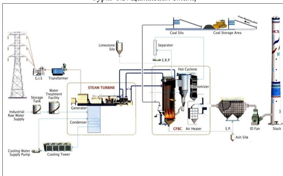
Зураг 1.6. Цахилгаан станцын технологийн схем
