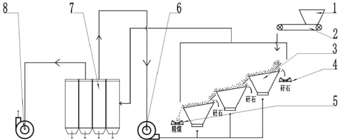
Зураг 1. Тоног төхөөрөмжийн холболтын зураг
