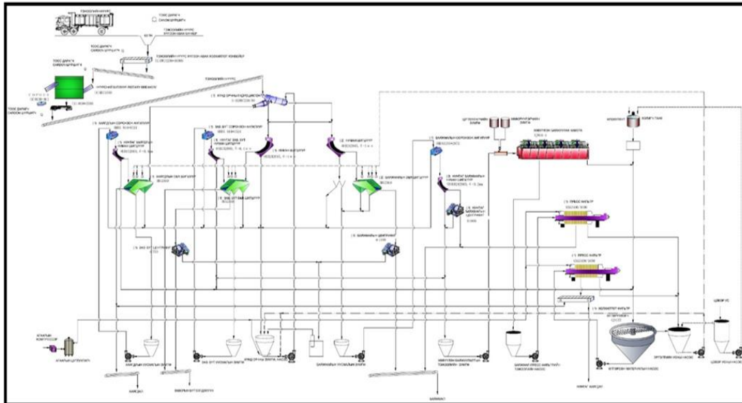
Нүүрс баяжуулах үйлдвэрийн технологийн схем
