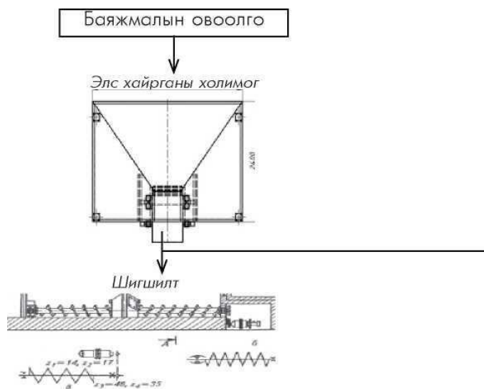
Зураг 6. Технологийн схем
