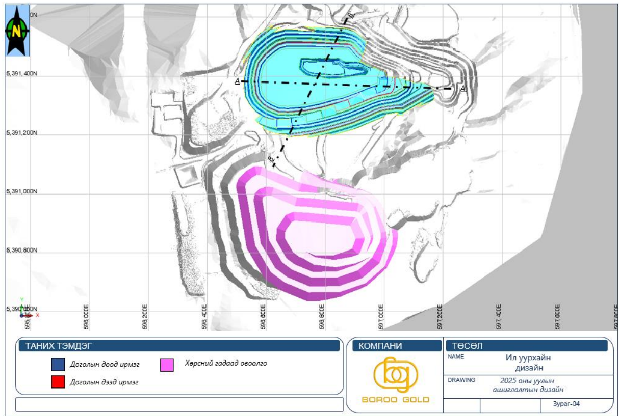
Зураг 4. Ил уурхайн овоолгын план зураг
