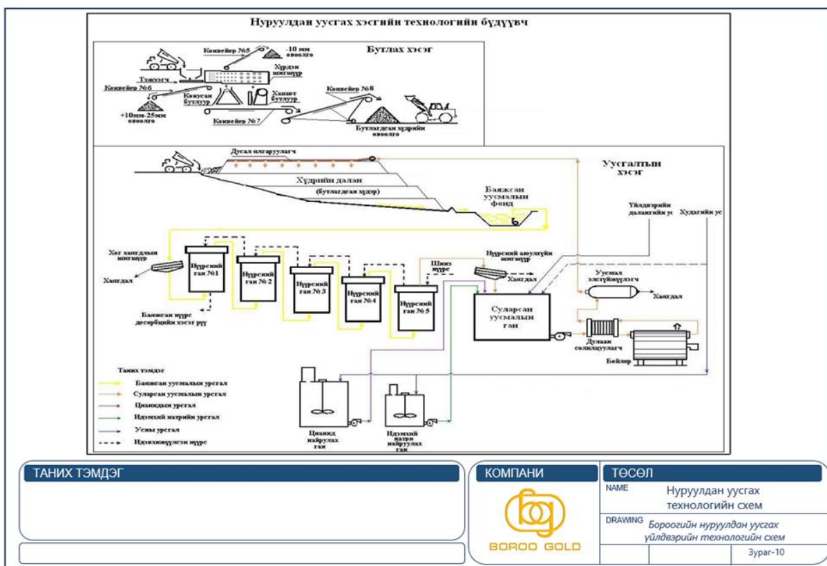
Зураг 3. Нуруулдан уусгах хэсгийн технологийн бүдүүвч
