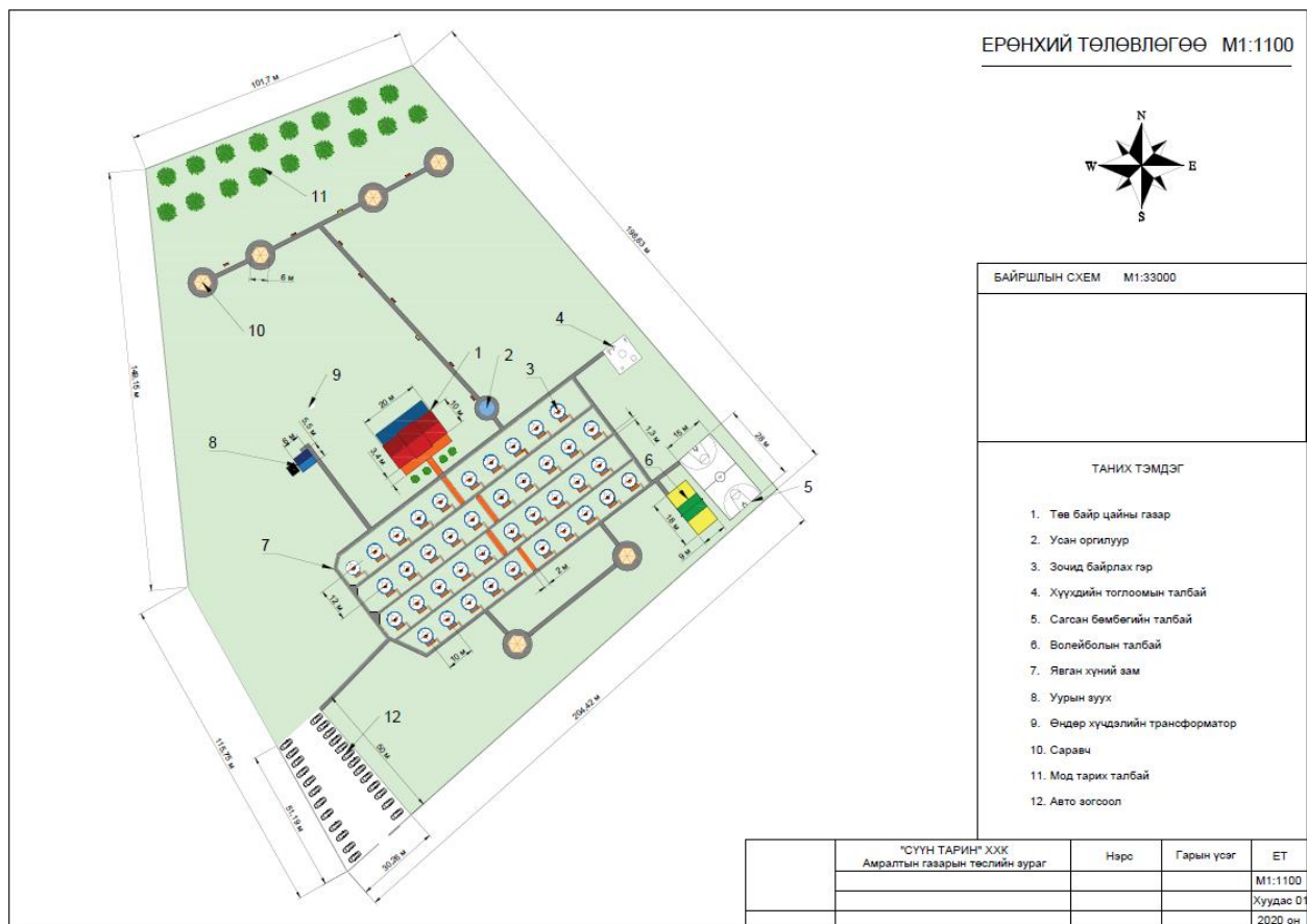
Зураг 1. Амралтын газрын зохион байгуулалт
