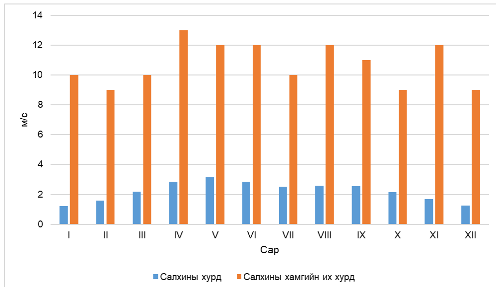
Зураг 10. Судалгааны талбайн орчны салхины хурд /Улаанбаатар станц 2005-2017/
