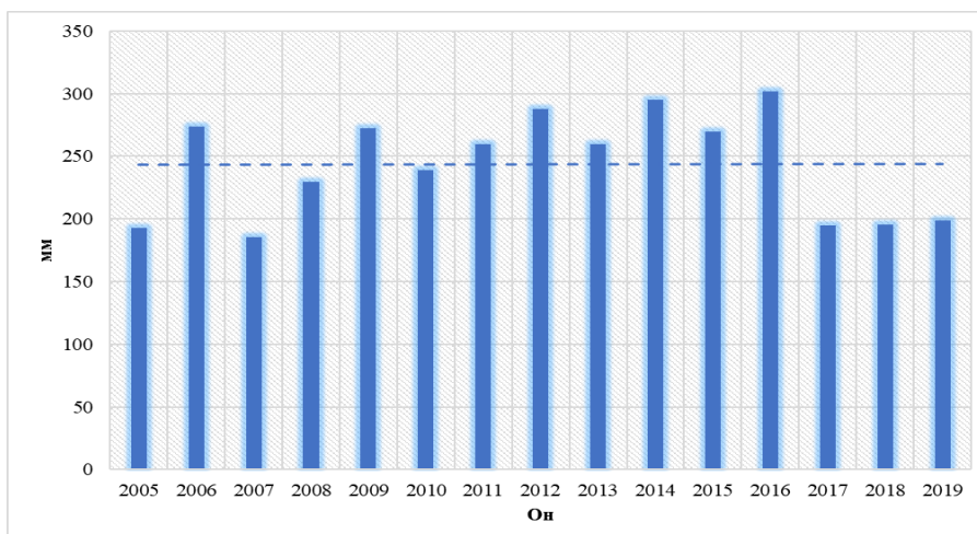
Зураг 9. Нийлбэр тунадас
