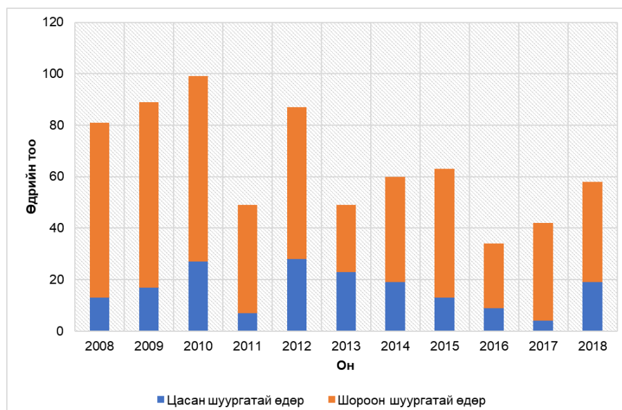
Зураг 11. Цасан болон шороон шуургатай өдрийн тоо
