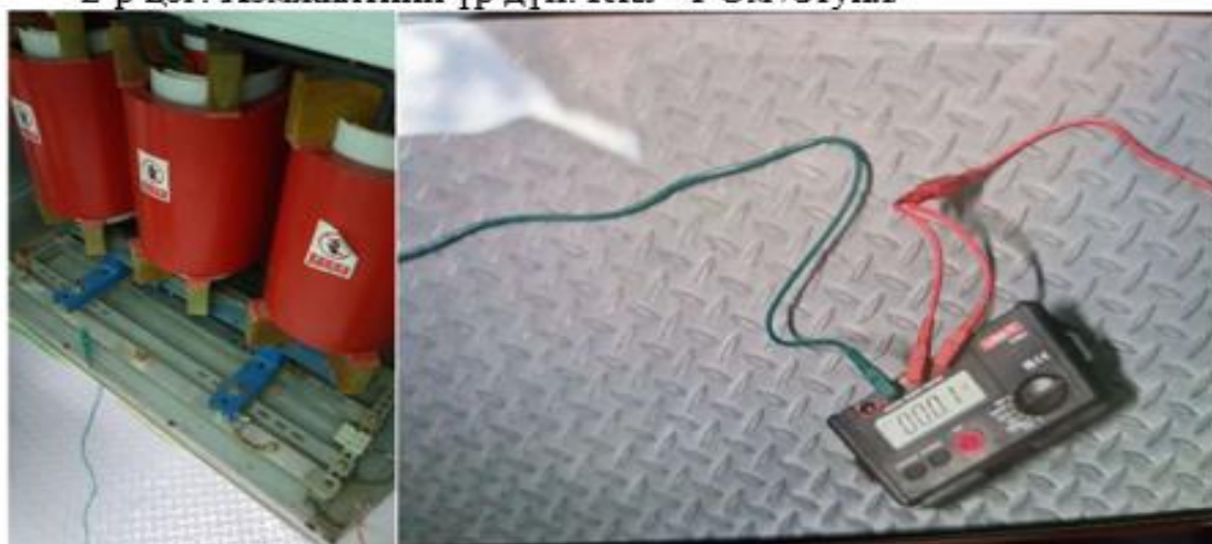
Зураг 2. 35кВ ХХБ газардуулгын хүрээний хэмжилт /1-р цэг/
