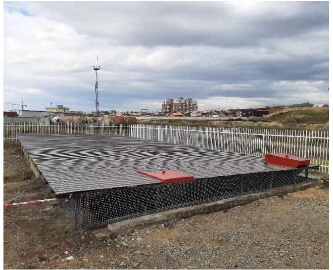
Зураг-2 Шатахуун хадгалах , түгээх хэсэг бетонон талбай далангийн зураг
