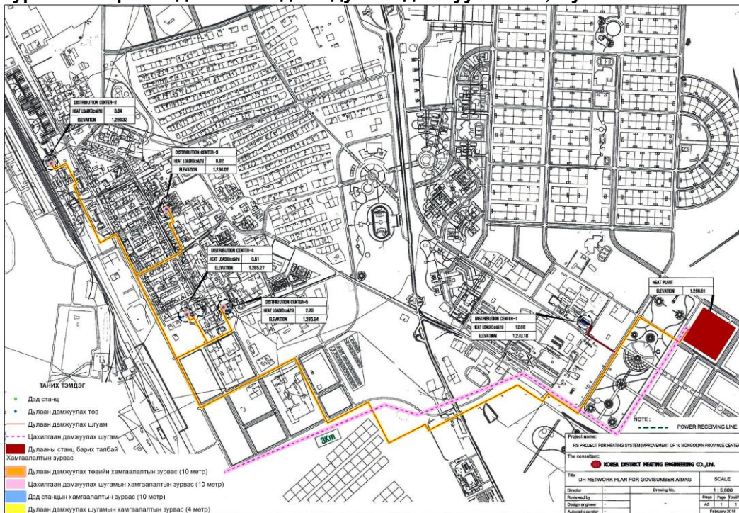
Зураг 4: Чойр хотод төлөвлөгдсөн дулаан дамжуулах төв, шугам хоолойн байршил
