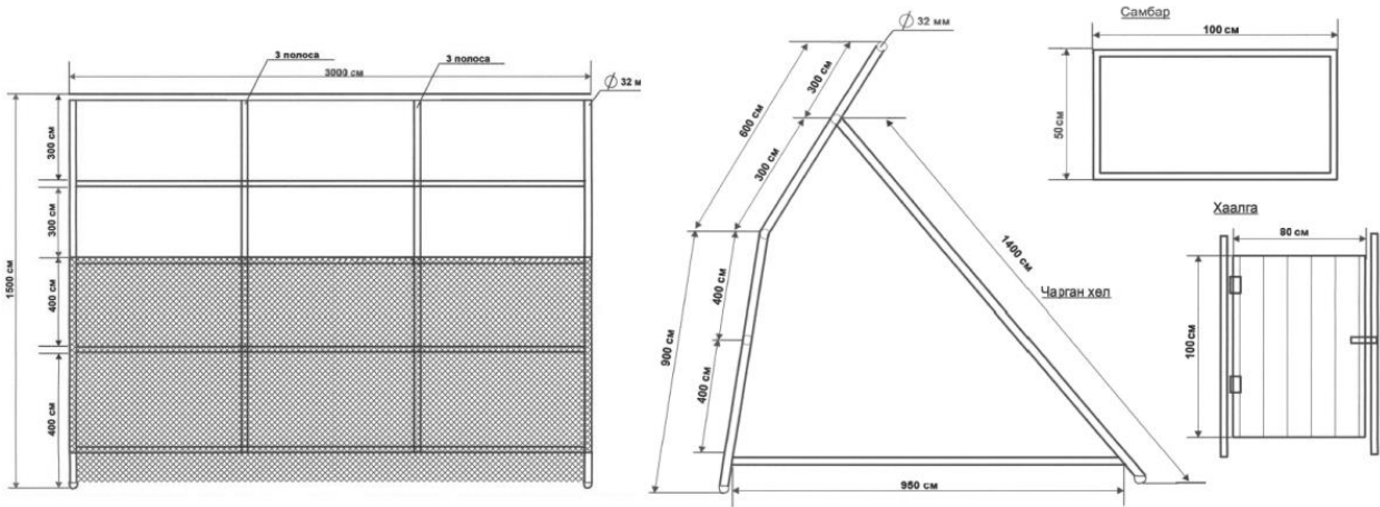
Зураг 7. Байгальд ээлтэй аргаар хашиж хамгаалах загвар гаргасан
