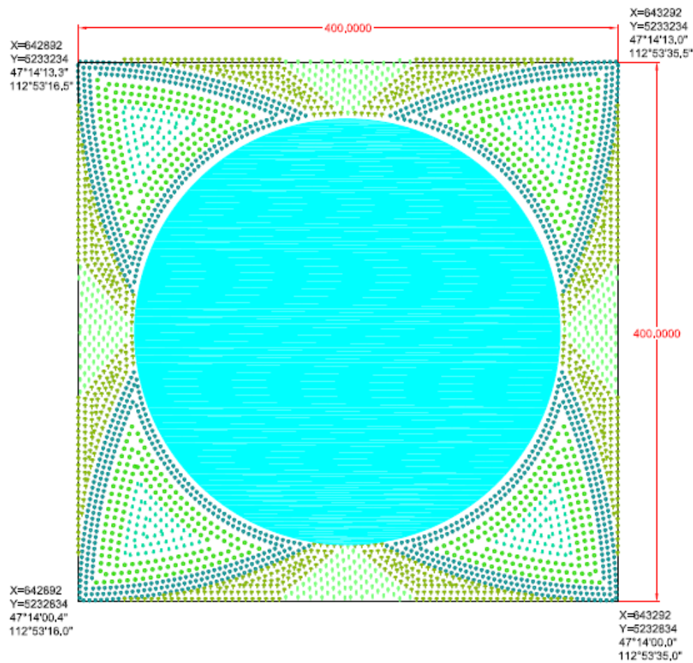
Зураг 15. Хөв цөөрмийн ерөнхий төлөвлөлт
