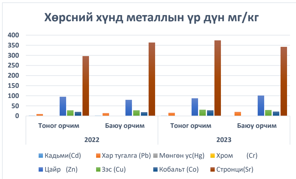
Зураг 16. Хөрсний хүнд металлын үр дүн мг/кг
