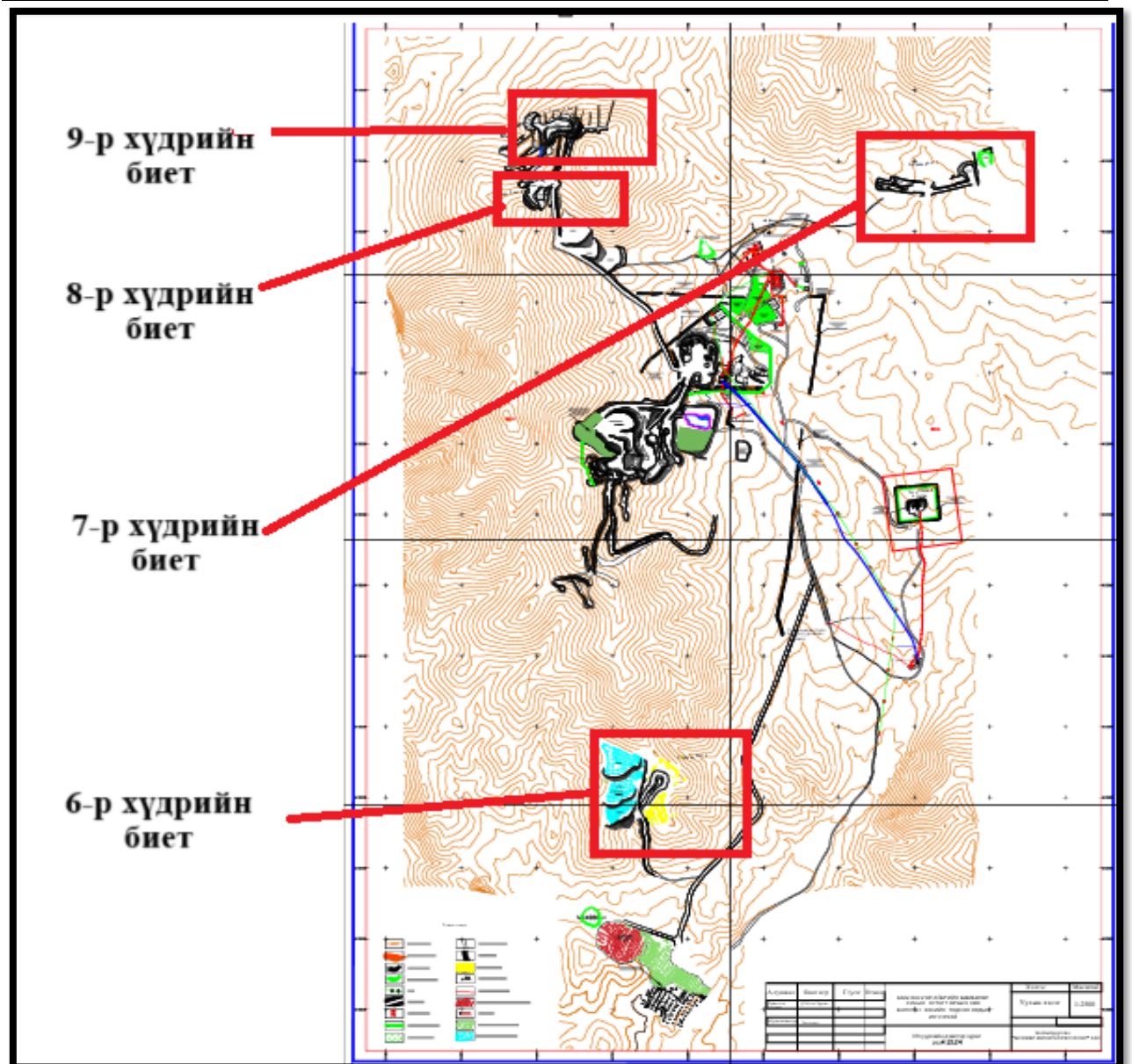
Зураг 3. Уулын ажлын зураг
