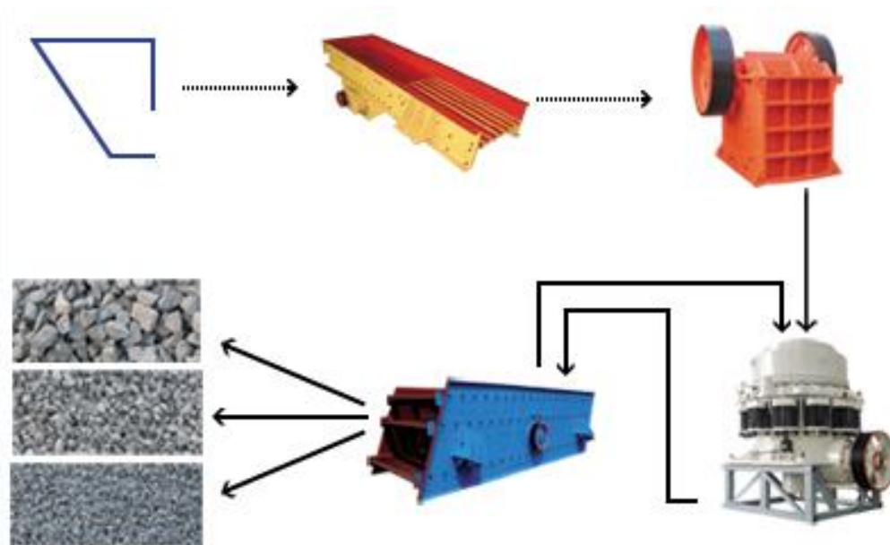
Зураг 2. Бутлан ангилах хэсгийн дамжлагын схем зураг
