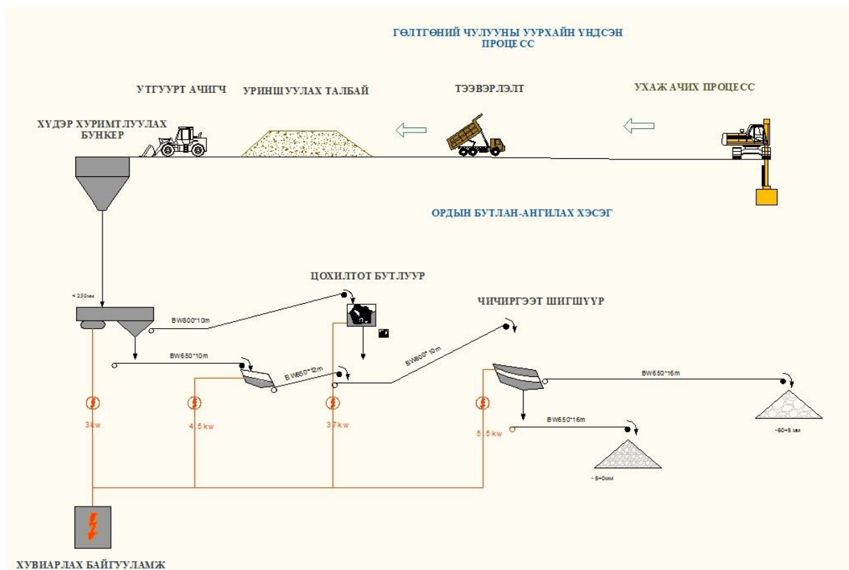
Тоног төхөөрөмжийн холболтын схем
