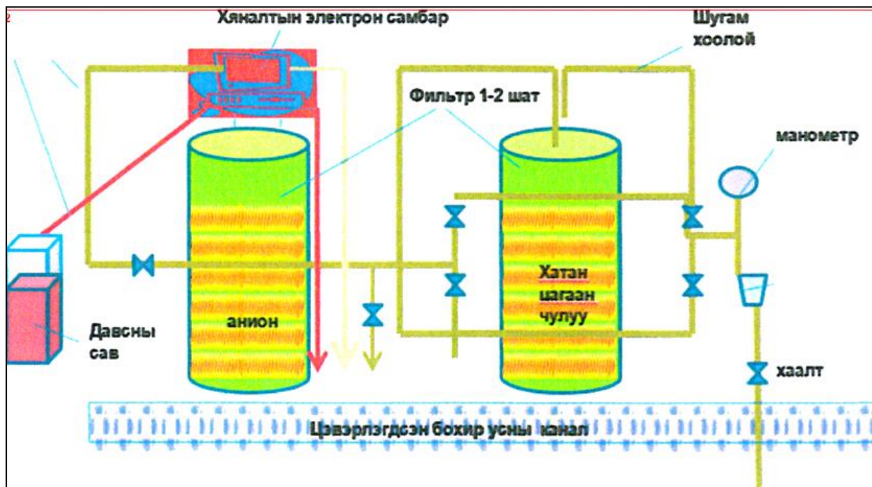
Зураг.17 Цэвэрлэх байгууламжийн схем
