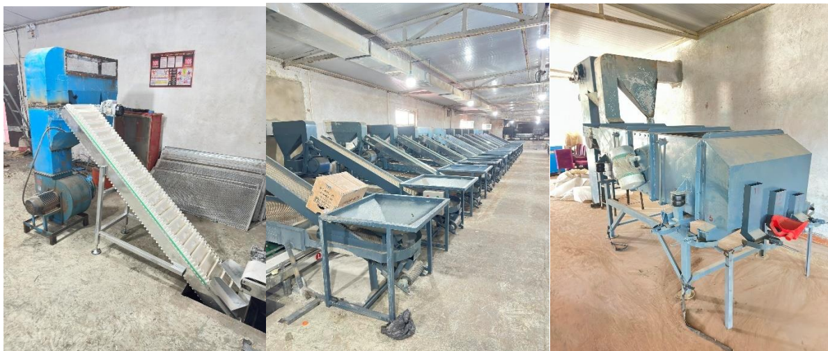
Зураг 10. Хальснаас ялгах машин
