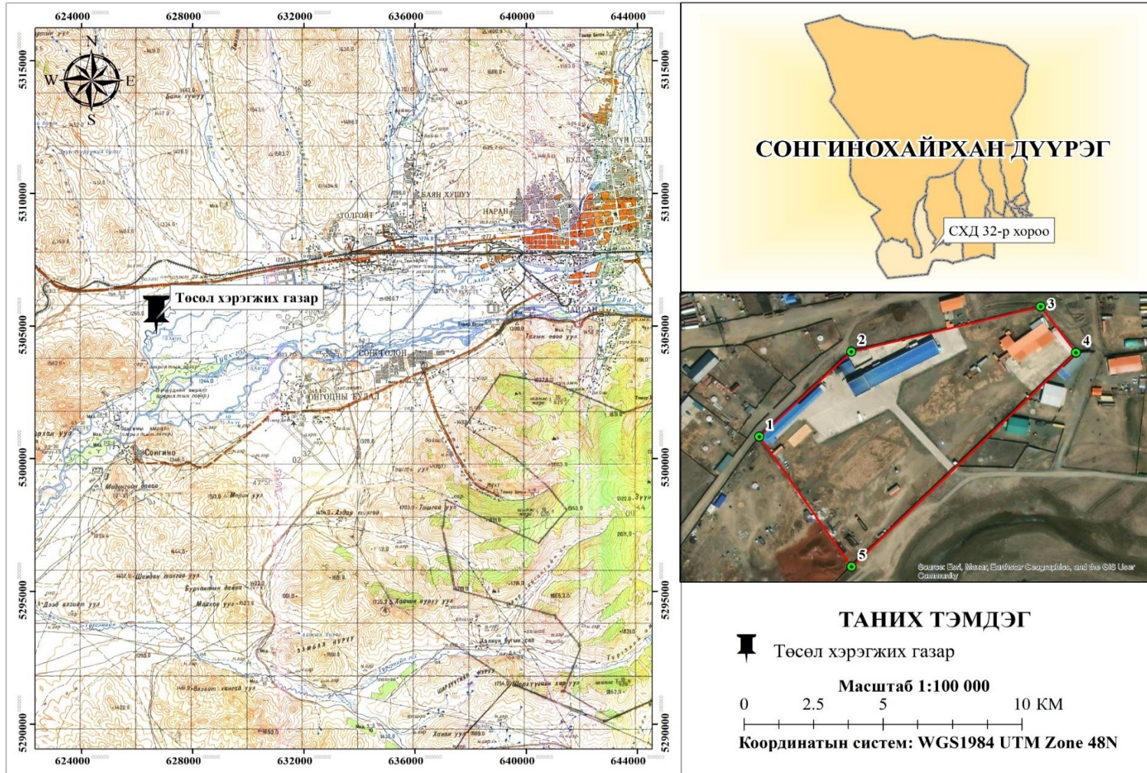
Зураг 2. Төслийн талбайн ерөнхий байрилын зураг
