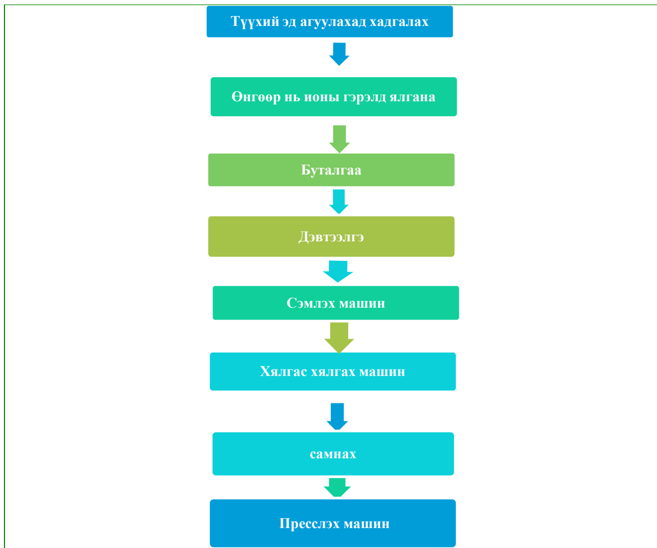
Ноос ноолуурын самнах үйлдвэрийн технологийн схем
