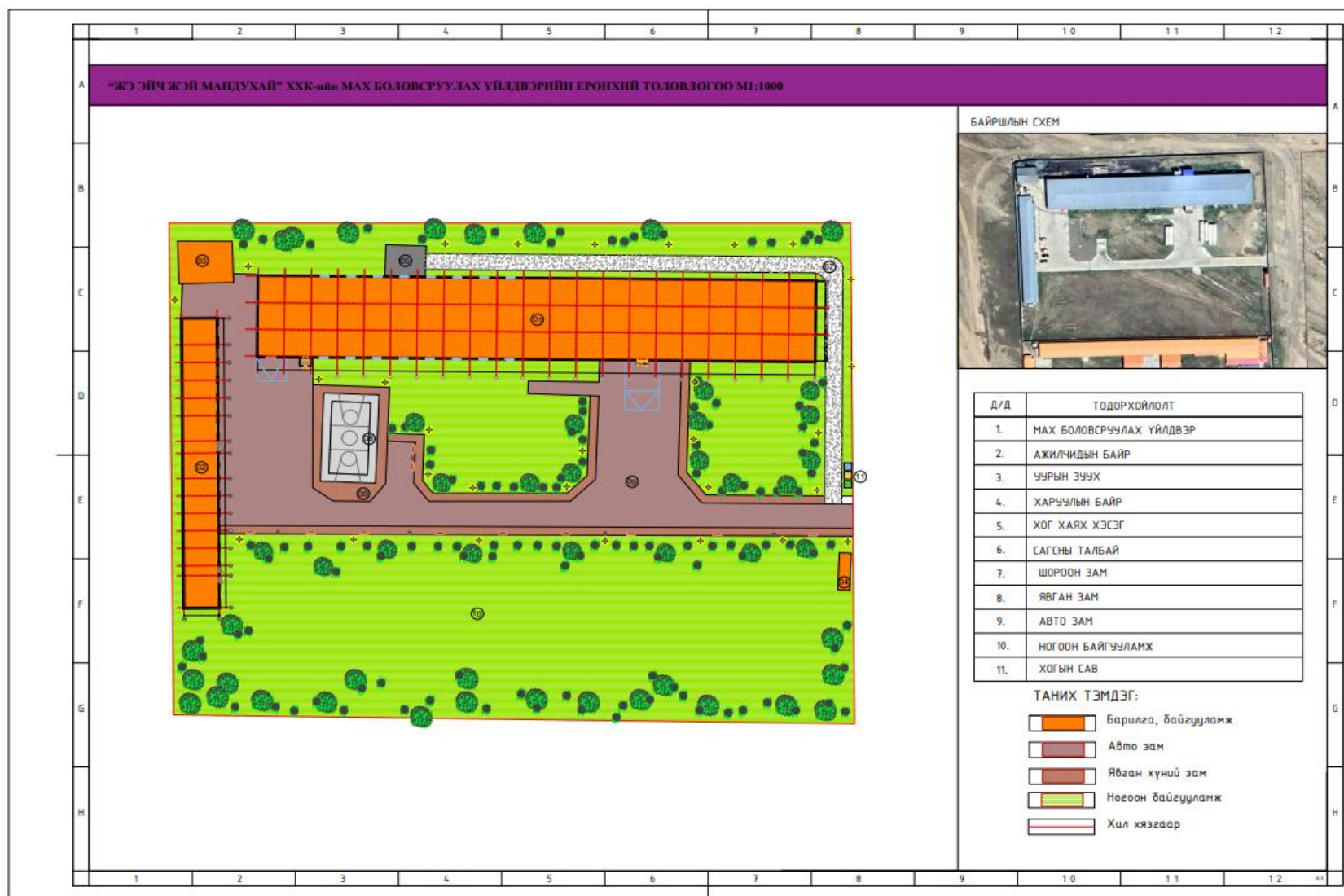
Зураг 1. “Дулааны аргаар мах боловсруулах үйлдвэр”-ийн ерөнхий төлөвлөлтийн зураг
