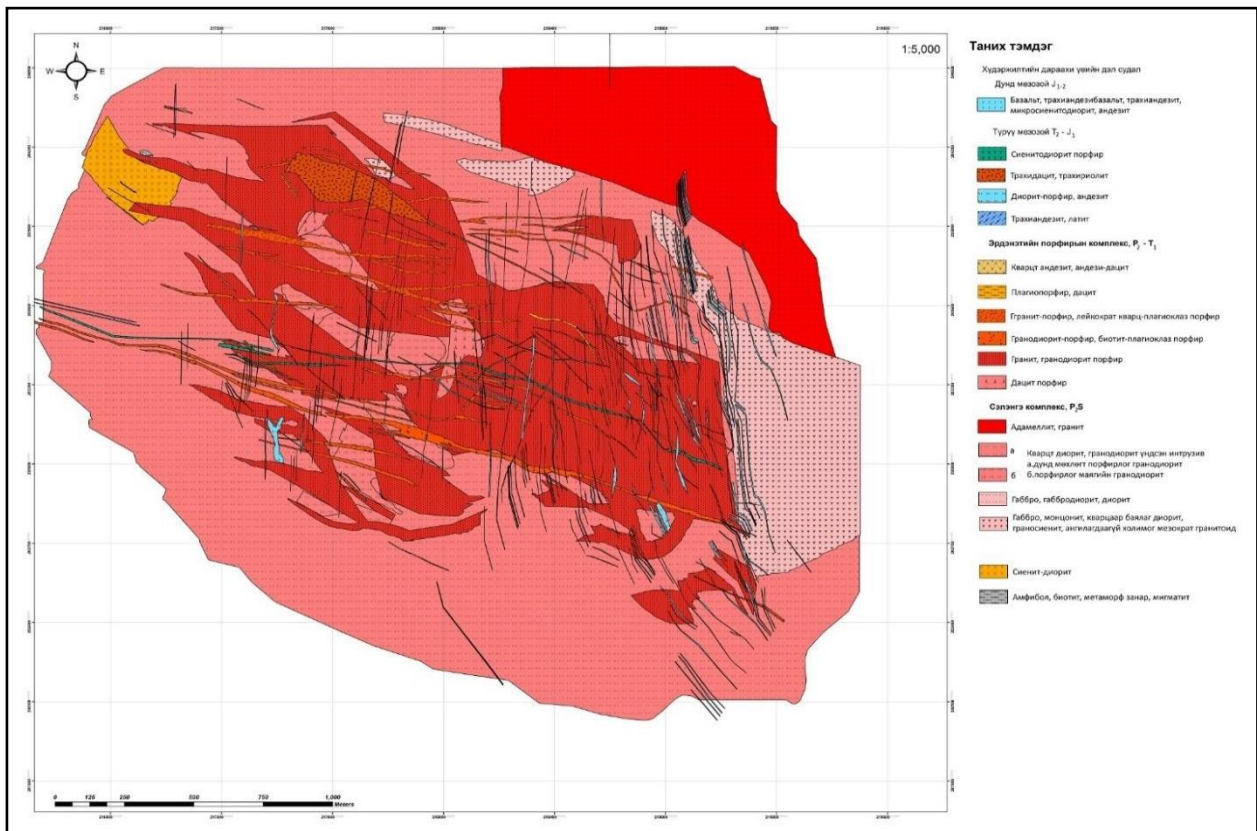
Зураг 6. Уурхайн “Баруун-Хойд” хэсгийн геологийн тогтоц
