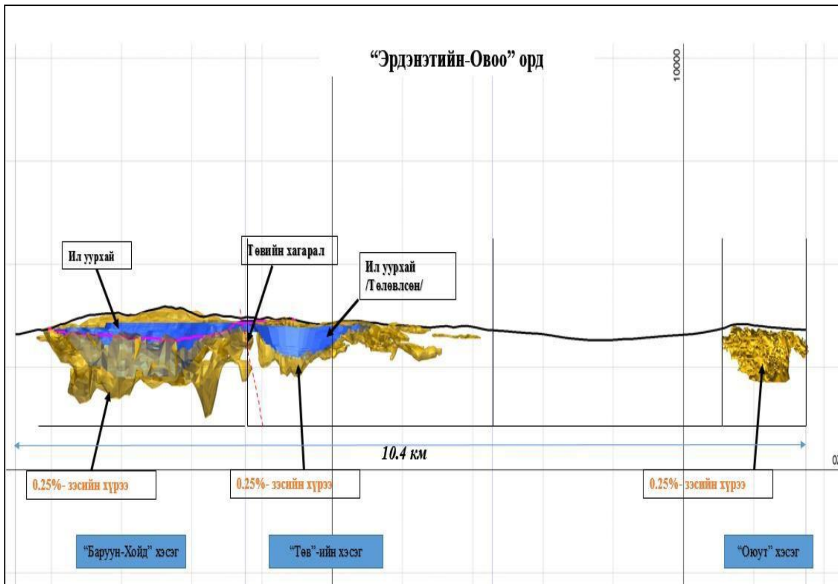
Зураг 7. Уурхайн ашигт малтмалын нөөцийн схем зураг
